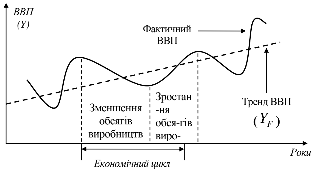
Рис. 1. Циклічні коливання на фоні довгострокового тренду
