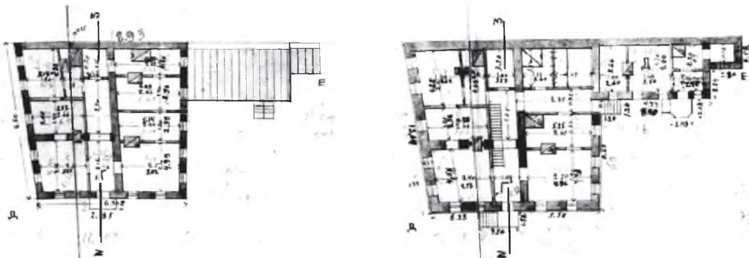
Іл. 9,10. Плани першого і другого поверхів житлового будинку «Г» і план першого поверху флігеля «Д», вул. Госпітальна, 1.
