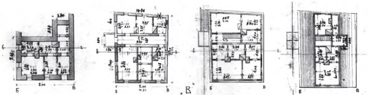
Іл.11,12,13,14. Плани цокольного, першого і другого поверхів та мансарди будинку «В», вул. Госпітальна (сьогодні втрачений).
