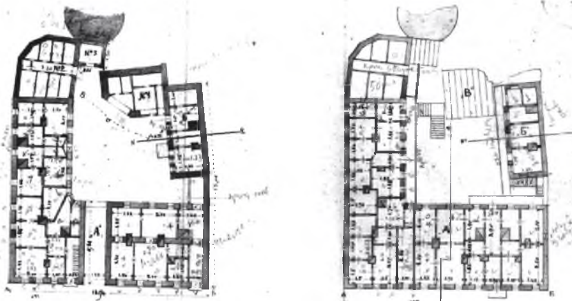
Іл. 7,8. Плани першого і другого поверхів житлового будинку «А» та плани двоповерхового флігеля «Б», вул. Госпітальна, 3.
