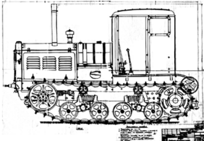
Іл. 5. Гусенічний трактор ХТЗ-НАТИ-ІТА. Вид збоку. 1941 р. (ЦДНТА України. Ф. Р-26. К. 2-151. Оп. 4. Од. зб. 25. Арк. 1)
