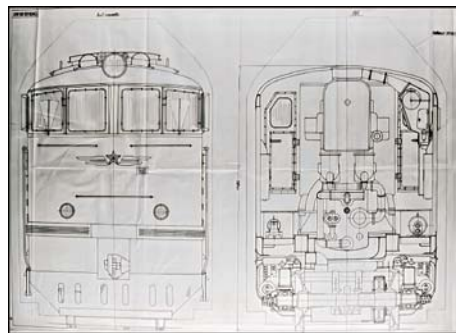
Іл. 4. Загальний вид тепловоза ТЕ100. Фрагмент кресленика. 1960 р. (ЦДНТА України. Ф. Р-25. К. 2-65. Оп. 9. Од. зб. 3262)
