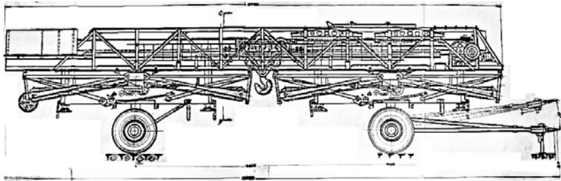
Іл. 6. Козловий кран 8Т21. Загальний вид. 1952 р. (ЦДНТА України. Ф. Р-50. К. 2-53. Оп. 1. Од. зб. 3. Арк. 7)
