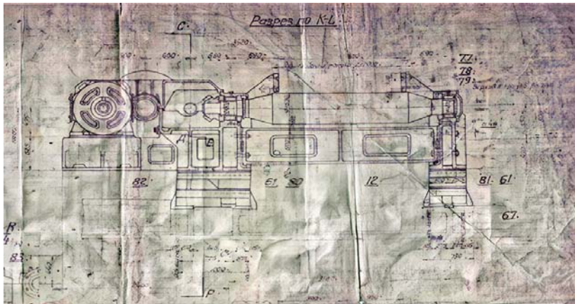
Іл. 2. Слябінг Ф1100 мм. Загальний вид робочого рольгангу. Фрагмент кресленника. 1935 р. (ЦДНТА України. Ф. Р-4. К. 2-55. Оп. 1. Од. зб. 1. Арк. 1)
