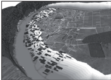
Рис. 2. 3D-модель максимального затоплення с. Горошова
