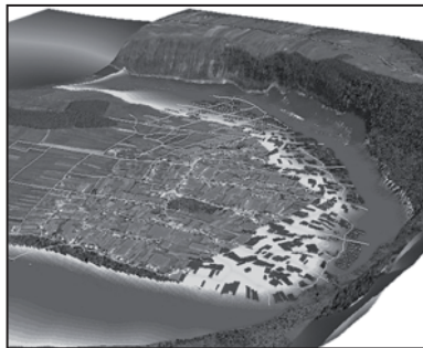
Рис. 2. 3D-модель максимального затоплення с. Горошова
