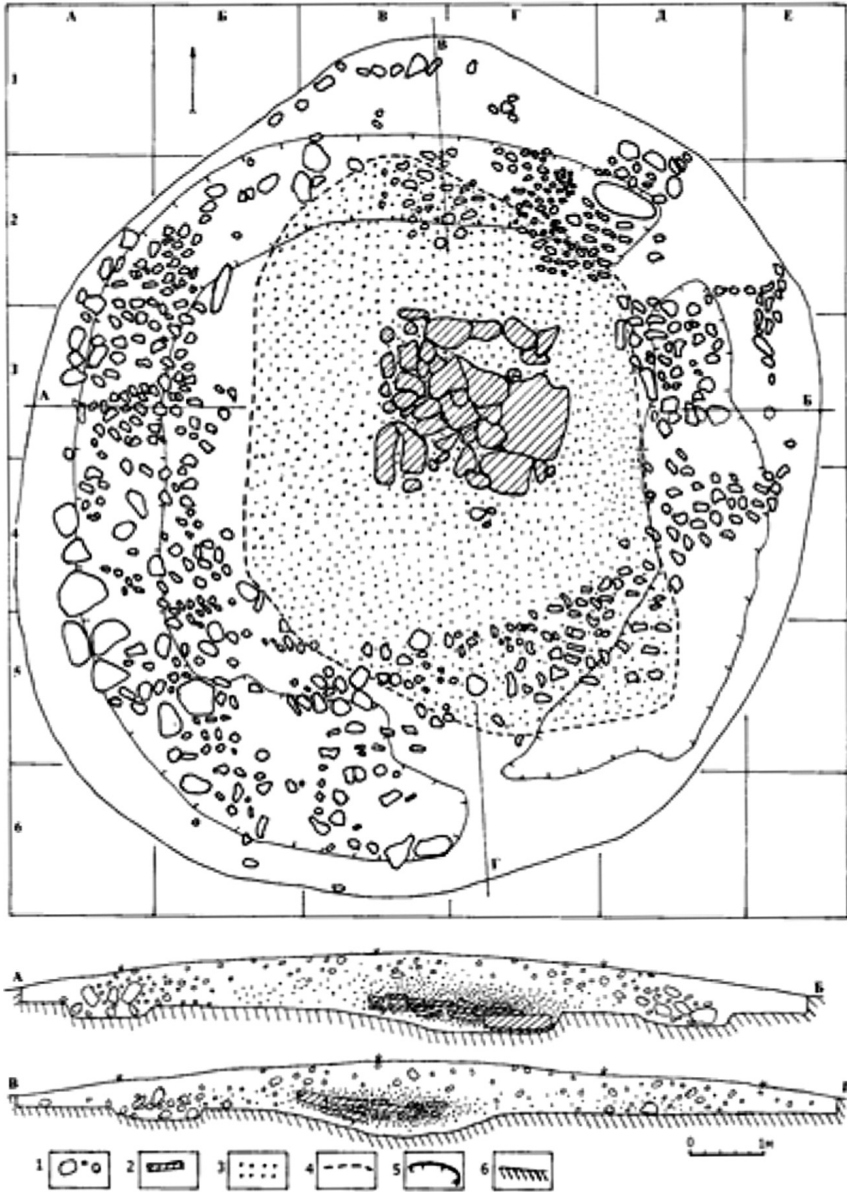
Рис. 1. План кургану № 1: 1 – каміння; 2 – кам'яна підлога; 3 – випалений ґрунт; 4 – межі проваленого шару; 5 – яма; 6 – материк
